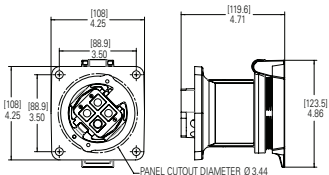
AR receptacle - spring door
